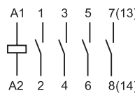
4 NO (4310)
